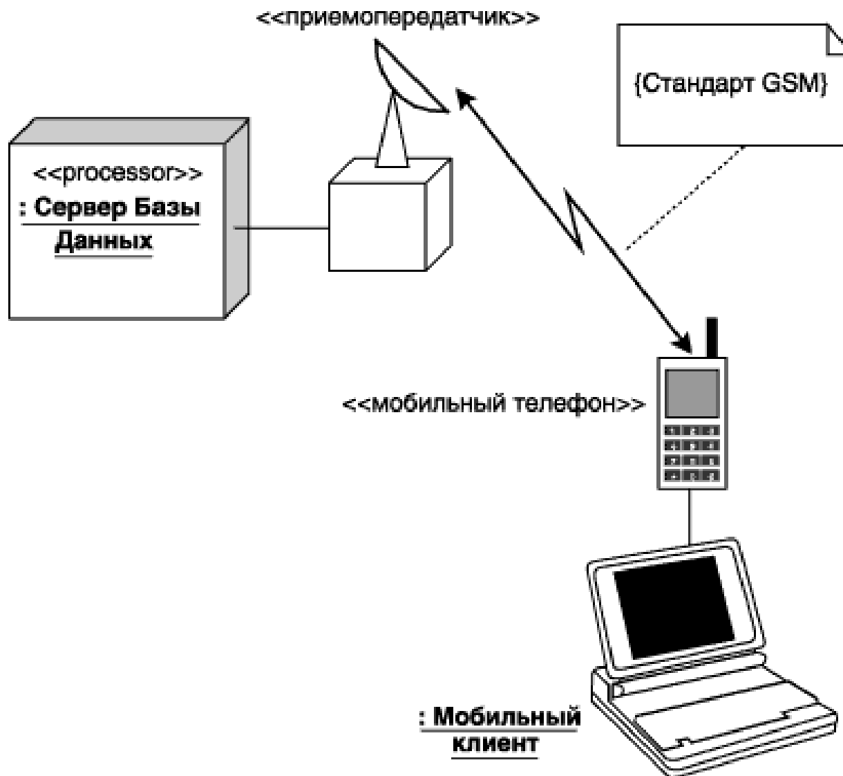
Диаграмма развертывания для системы мобильного доступа к корпоративной базе данных
